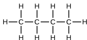
n -butane
