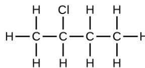
2-chlorobutane
